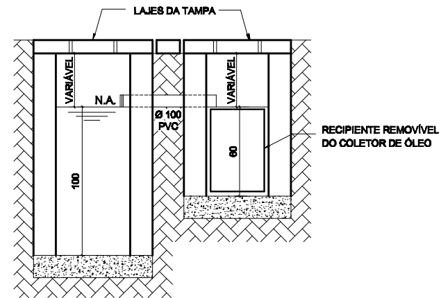
CORTE B-B SEM ESCALA
